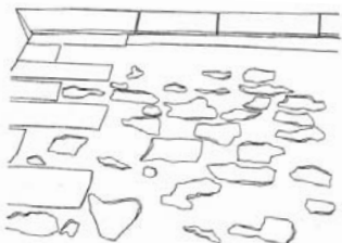
La finition de la façade doit être plane pour laisser la pluie glisser et ne pas accrocher les poussières. Très peu de moellons doivent apparaître
