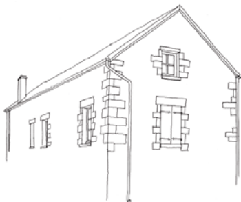
Une fenêtre en pignon, désaxée du faîtage, alignée sur celle de l'étage, permet d'éclairer le comble en encuvement
