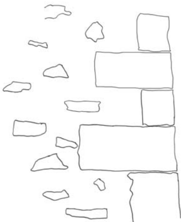
Harpe en pierre de taille d'un mur en moellon calcaire et grès
