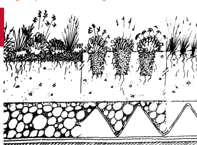
Source : toits et murs végétaux, Nigel Dunnnett et Noël Kingsbury, édition du Rouergue
