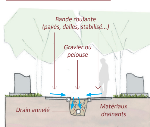
COUPE SUR TRANCHÉE DRAINANTE
