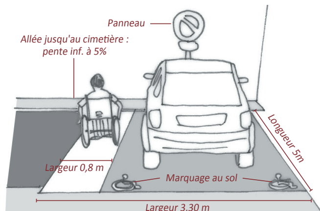
SCHÉMA INDICATIF / STATIONNEMENT
