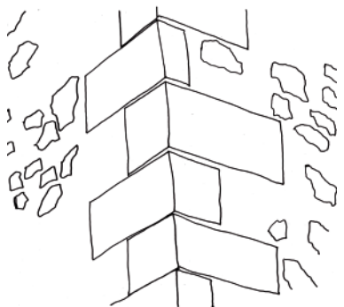
Chaînage d'angle en pierres de taille harpées sur un mur de moellon enduit
