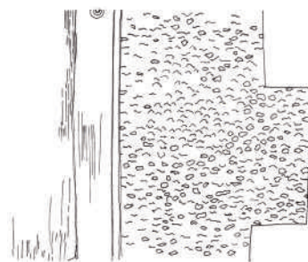
Détails d'un enduit tyrolien avec modénature en enduit lissé
