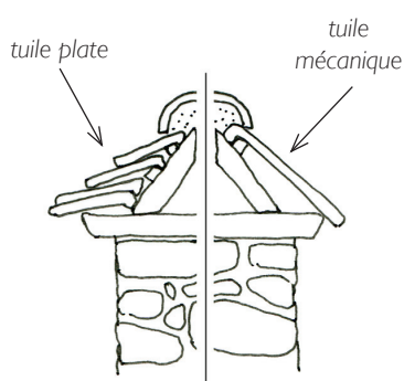
Chaperon en tuile à deux versants
