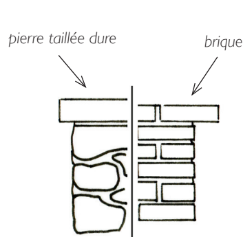
Couronnement plat
